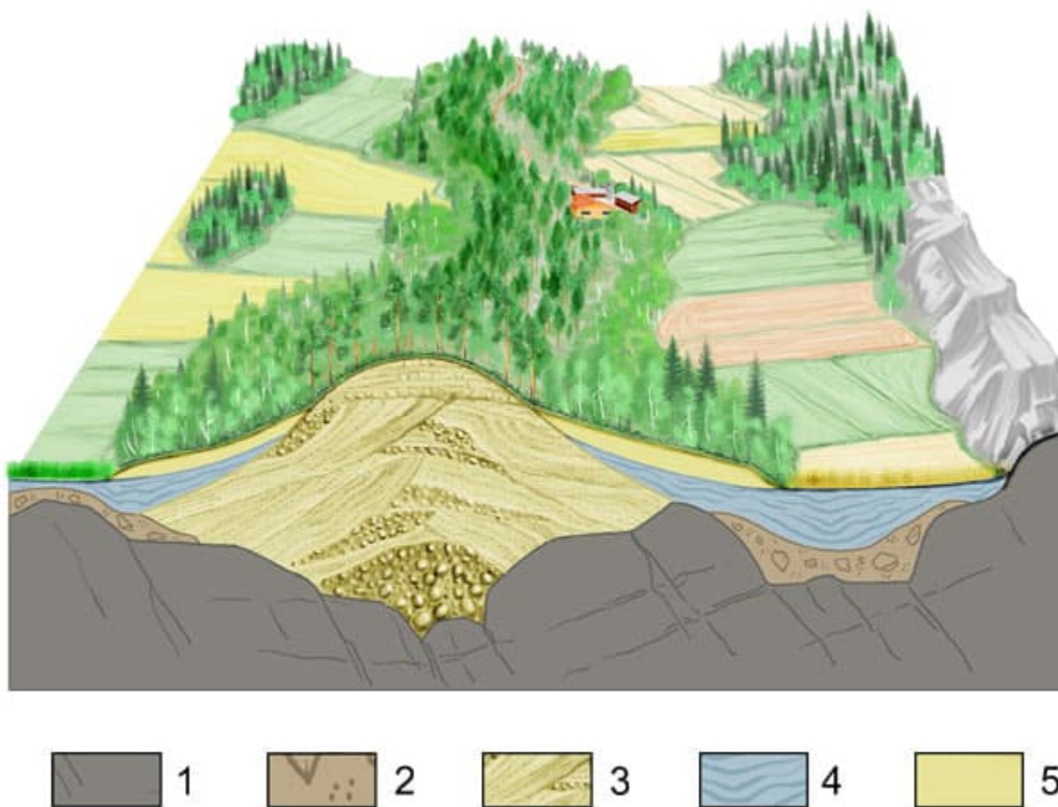
Kuva 1. Harjun poikkileikkaus. 1. Kallio, 2. Pohjamoreeni, 3. Harjuaines (sora ja hiekka), 4. Savi ja siltti, 5. Rantakerrostuma (hiekkä) (geologia.fi 2018)
