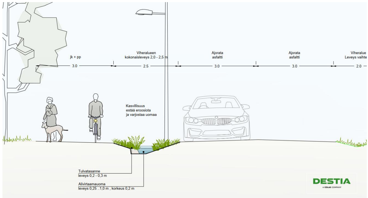
Kuva 16. Esimerkkipoikkileikkaus Teollisuustien tulevasta tilanteesta, jossa hulevesiä ohjataan erotuskaistalle toteutettavaan avo-ojaan.
