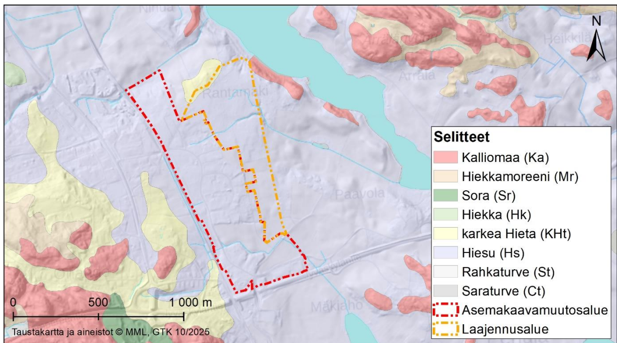
Kuva 8. Alueen maaperä GTK:n maaperäkartan 1:20 000 perusteella © Geologian tutkimuskeskus 2025.
