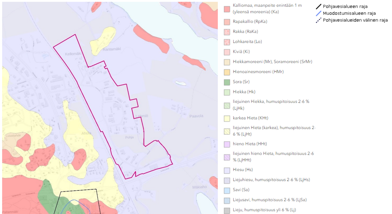
Kuva 9. Ote suunnittelualueen maaperäkartasta (GTK) sekä pohjavedestä (Syke). GTK:n maaperäkartan mukaan suunnittelualueen maaperä on hiesua. Suunnittelualueen raja on osoitettu pinkillä viivalla.
