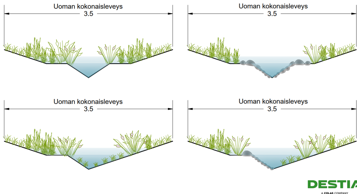
Kuva 17. Esimerkkejä erotuskaistan avo-ojan poikkileikkauksesta pohjapadon yläpuolisen levennyksen kohdalla, jossa hulevedet nousevat rankkasateen aikana ns. tulvahyllylle. Tulvahylly lisää ojan viivytyskapasiteettia. Kasvillisuus tai/ja kiveys estävät uoman pohjan ja luiskien eroosiota.
